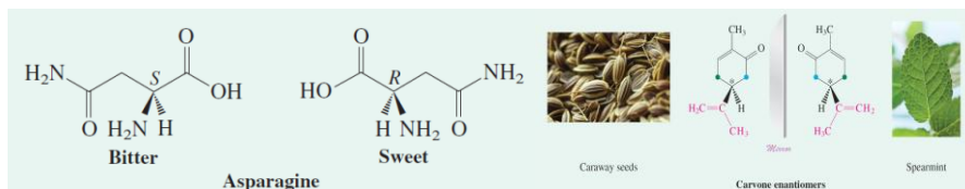
شکل ۱: انانتیومر
